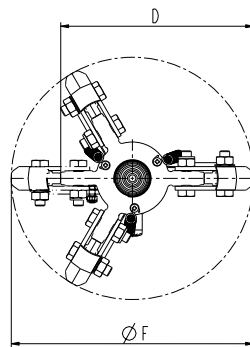
Måttskiss AH50/110
